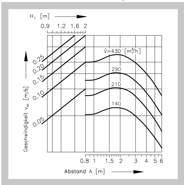
Diagramm 11 Einreihige oder mehrreihige Anordnung der Dralldurchlässe, wenn B ≥ 4 m
