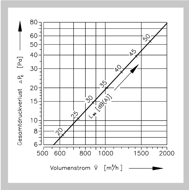
Diagramm 25. Druckverlust und Schalleistung
