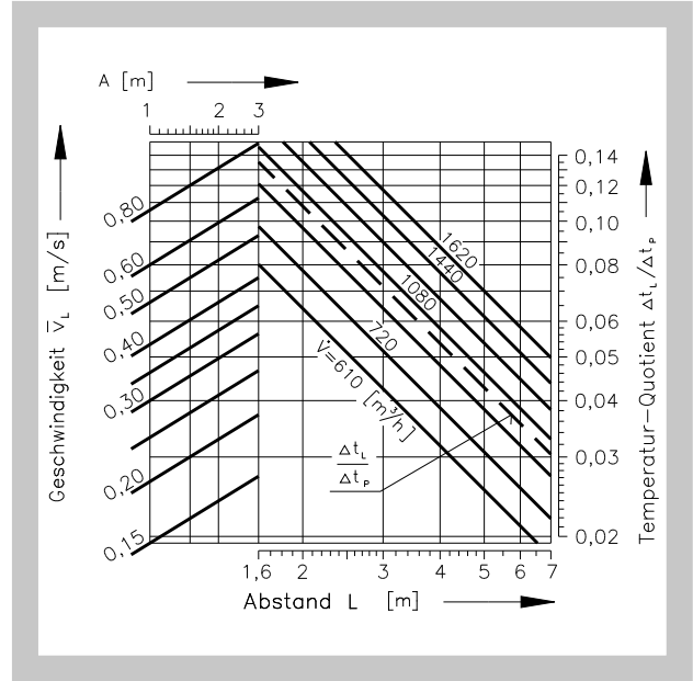
Diagramm 26 Luftgeschwindigkeit und Temperaturdifferenz
