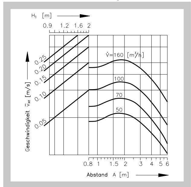
Diagramm 4 Mehrreihige Anordnung der Dralldurchlässe, wenn B = 3 m
