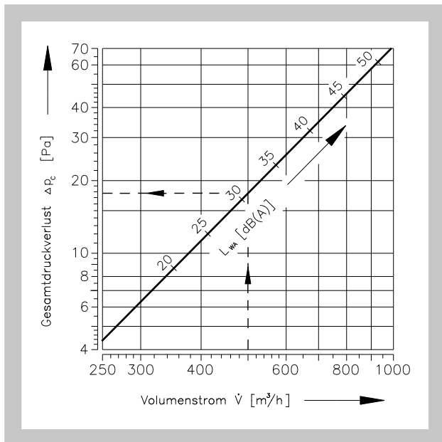
Diagramm 13 Druckverlust und Schalleistung
