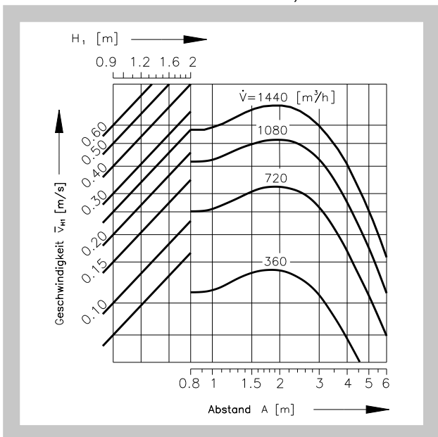
Diagramm 23 Einreihige oder mehrreihige Anordnung der Dralldurchlässe, wenn B ≥ 4 m
