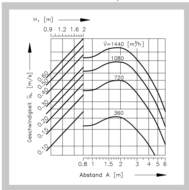
Diagramm 24 Mehrreihige Anordnung der Dralldurchlässe, wenn B = 3 m
