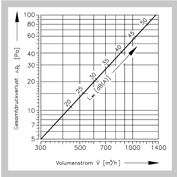
Diagramm 17 Druckverlust und Schalleistung
