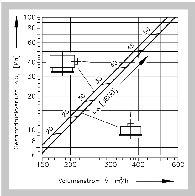
Diagramm 5 Druckverlust und Schalleistung
