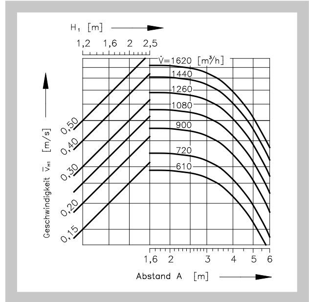
Diagramm 28 Mehrreihige Anordnung der Dralldurchlässe, wenn B = 3 m
