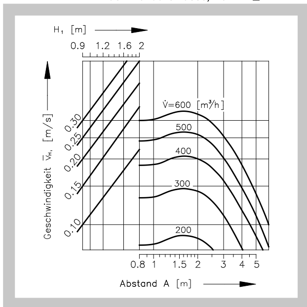
Diagramm 15 Einreihige oder mehrreihige Anordnung der Dralldurchlässe, wenn B ≥ 4 m
