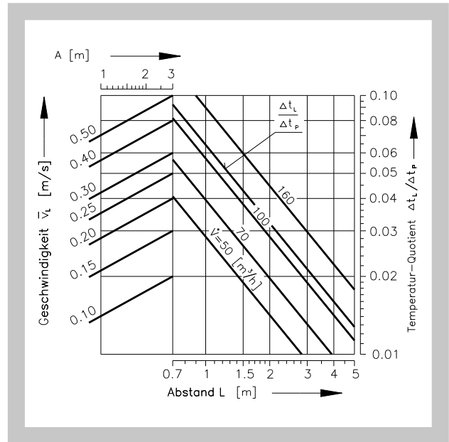
Diagramm 2 Luftgeschwindigkeit und Temperaturdifferenz
