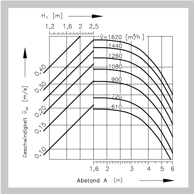
Diagramm 27 Einreihige oder mehrreihige Anordnung der Dralldurchlässe, wenn B ≥ 4 m
