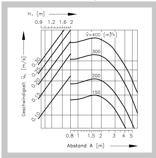
Diagramm 8 Mehrreihige Anordnung der Dralldurchlässe, wenn B = 3 m
