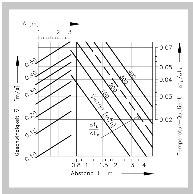
Diagramm 6 Luftgeschwindigkeit und Temperaturdifferenz
