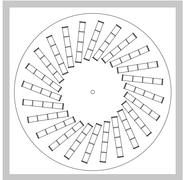
Abb. 4 Ausführung VVM/K - Runde Frontplatte
