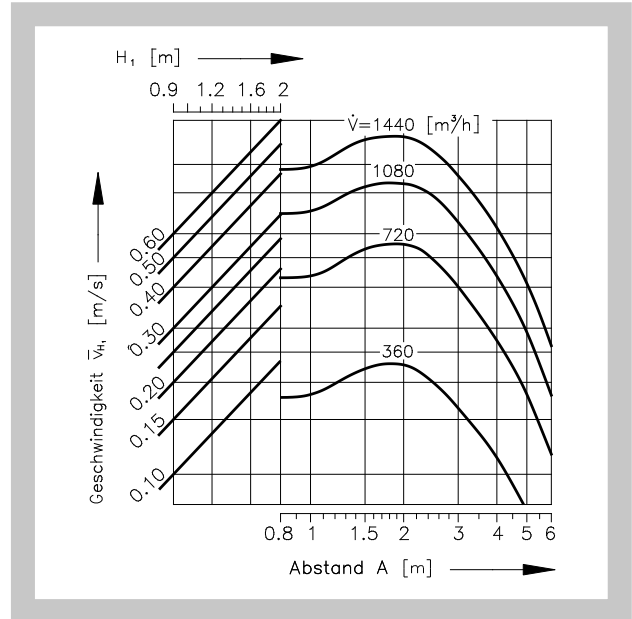
Diagramm 20 Mehrreihige Anordnung der Dralldurchlässe, wenn B = 3 m
