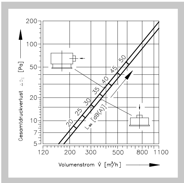
Diagramm 9 Druckverlust und Schalleistung
