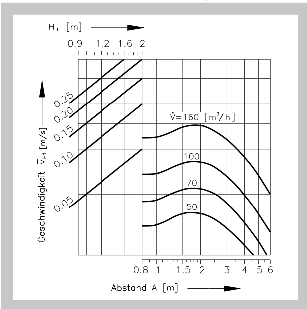
Diagramm 3 Einreihige oder mehrreihige Anordnung der Dralldurchlässe, wenn B ≥ 4 m
