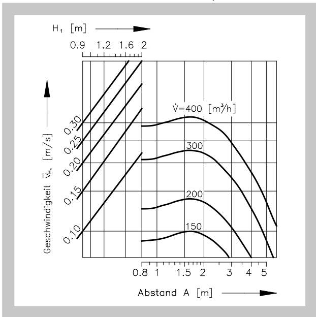
Diagramm 7 Einreihige oder mehrreihige Anordnung der Dralldurchlässe, wenn B ≥ 4 m
