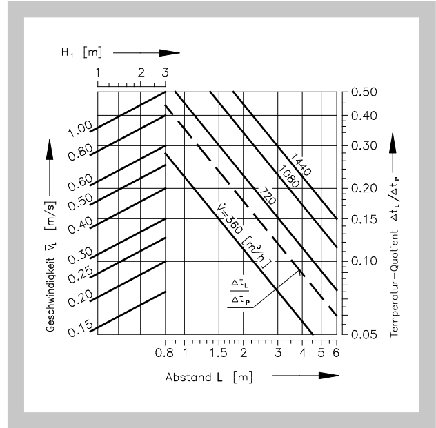
Diagramm 18 Luftgeschwindigkeit und Temperaturdifferenz
