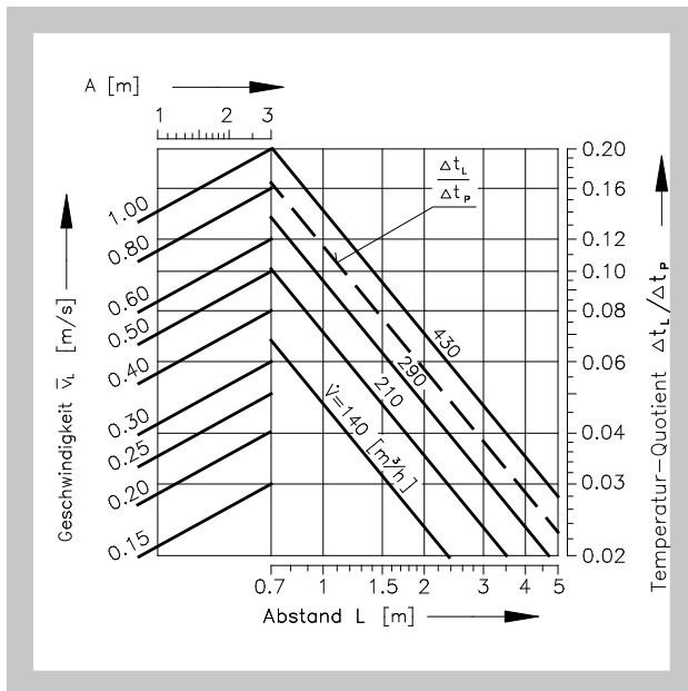
Diagramm 10 Luftgeschwindigkeit und Temperaturdifferenz
