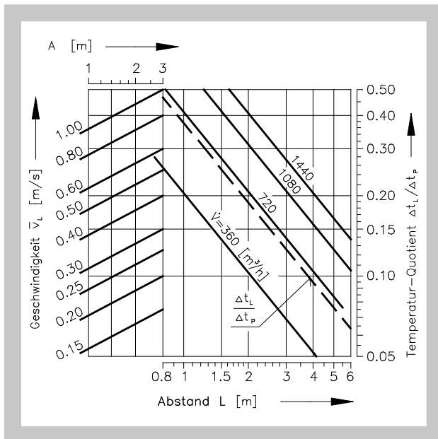
Diagramm 22 Luftgeschwindigkeit und Temperaturdifferenz
