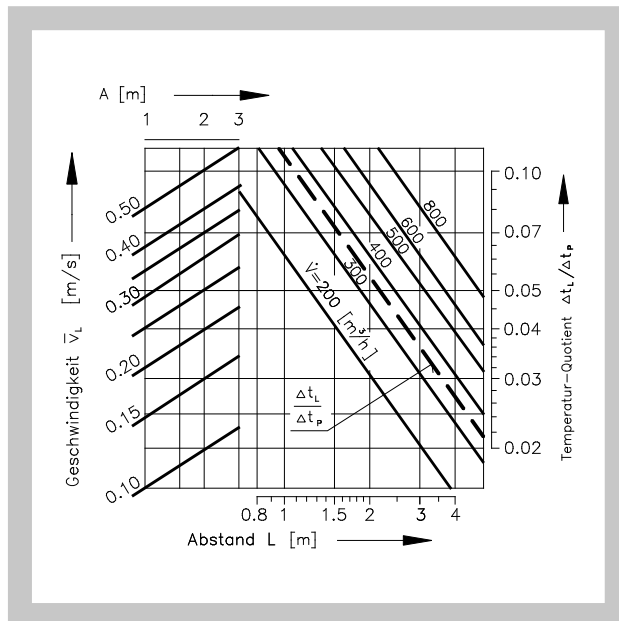
Diagramm 14 Luftgeschwindigkeit und Temperaturdifferenz
