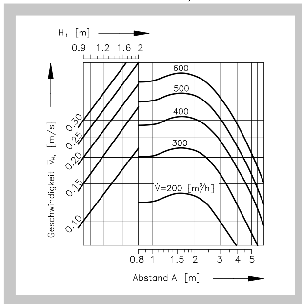
Diagramm 16 Mehrreihige Anordnung der Dralldurchlässe, wenn B = 3 m
