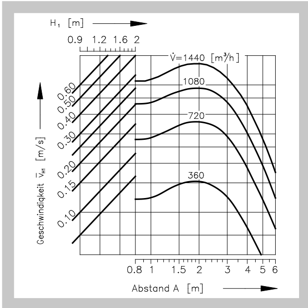
Diagramm 19 Einreihige oder mehrreihige Anordnung der Dralldurchlässe, wenn B ≥ 4 m
