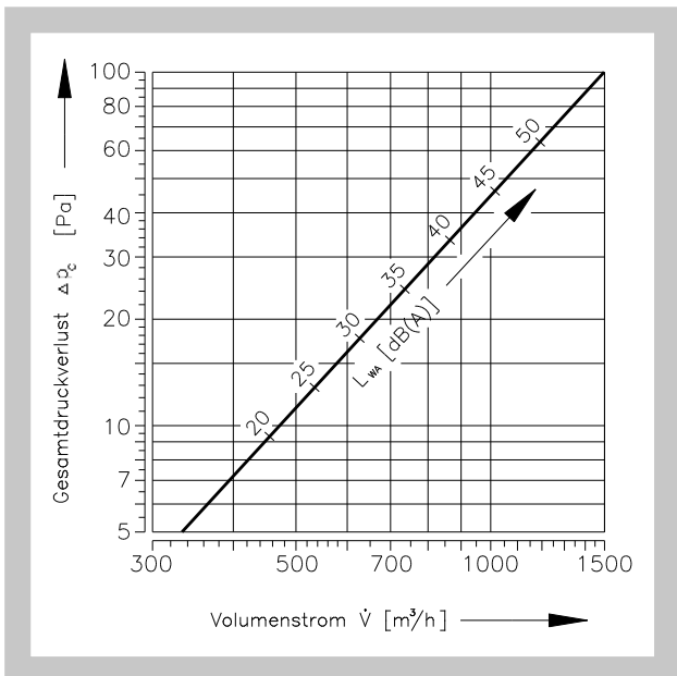
Diagramm 21 Druckverlust und Schalleistung
