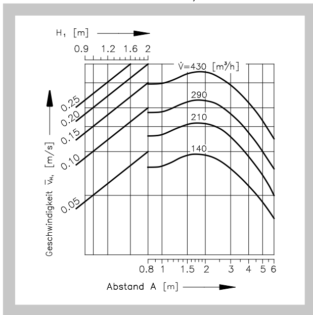
Diagramm 12 Mehrreihige Anordnung der Dralldurchlässe, wenn B = 3 m
