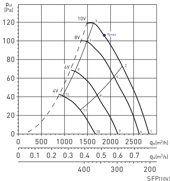
HXBR-300 ECOWATT
