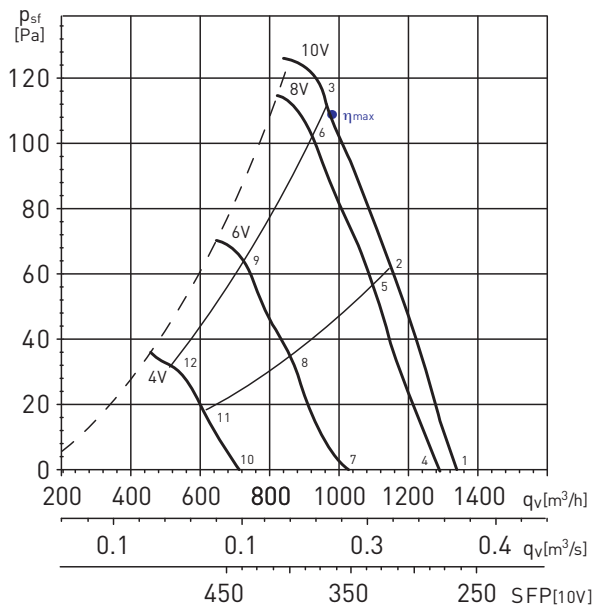
HXBR-200 ECOWATT
