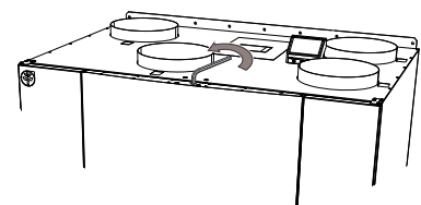
Bild 3 Öffnung der Frontklappe
