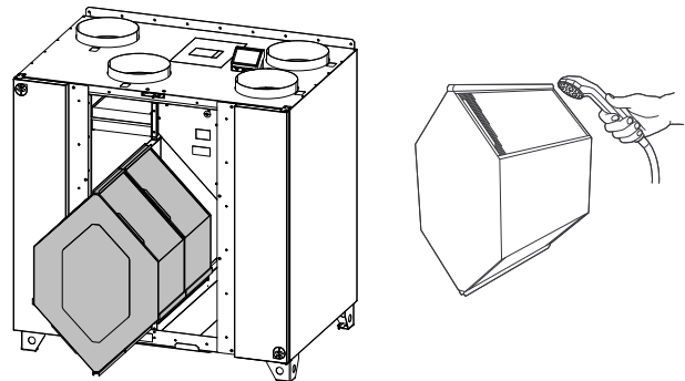
Bild 5 Entfernen und Reinigen des Wärmetauschers
