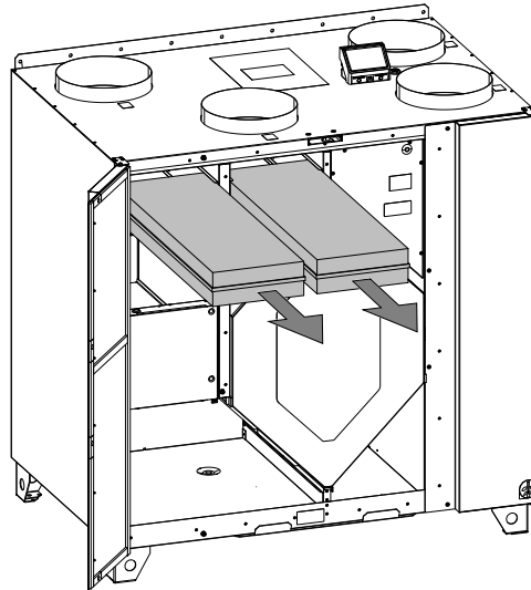
Bild 4 Auswechseln der Filter
