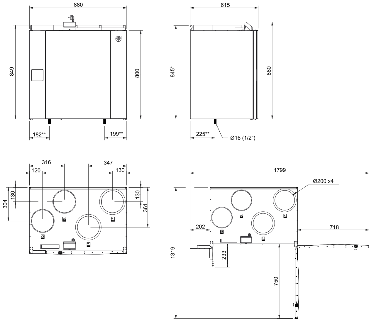
Bild 2 Abmessungen des linksseitigen Geräts
