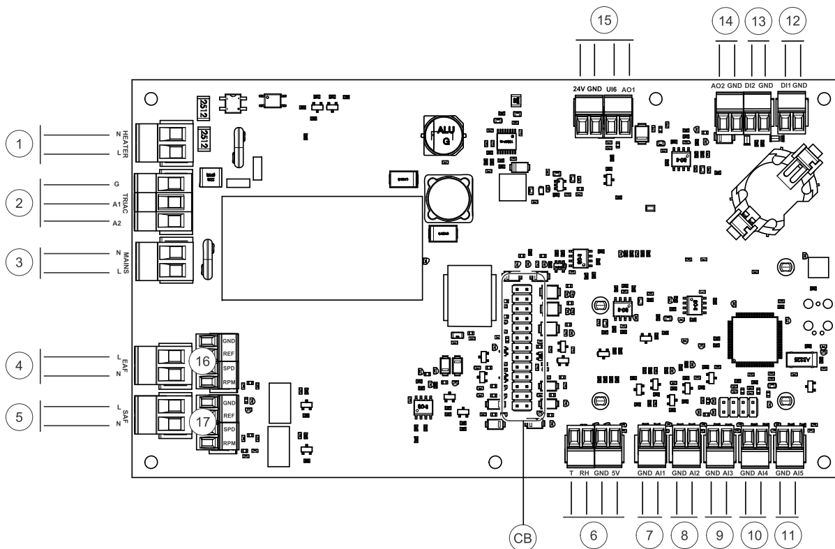
Bild 5 Anschlüsse der Hauptplatine
