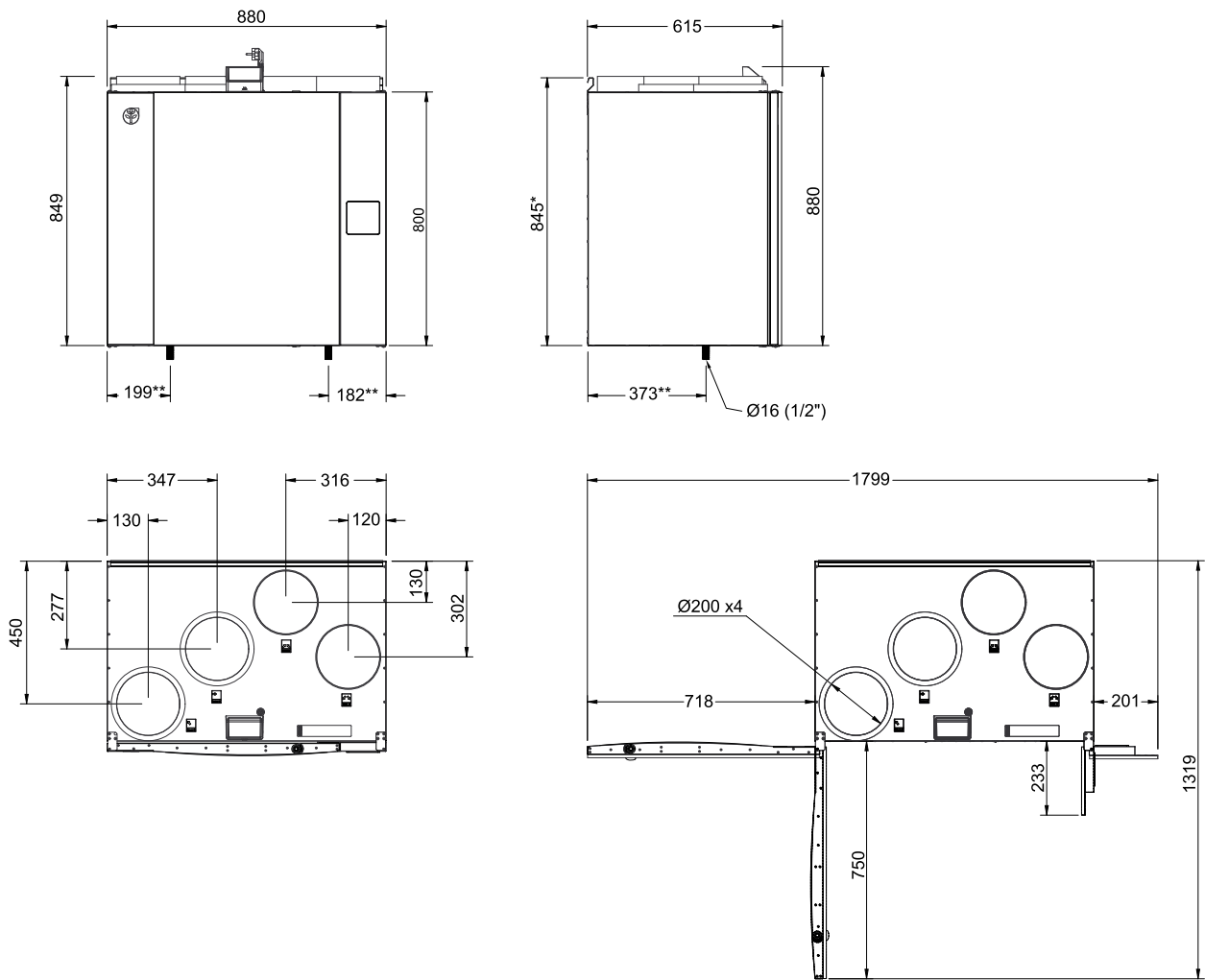
Bild 3 Abmessungen des Gerätes der Ausführung Zuluft rechts
