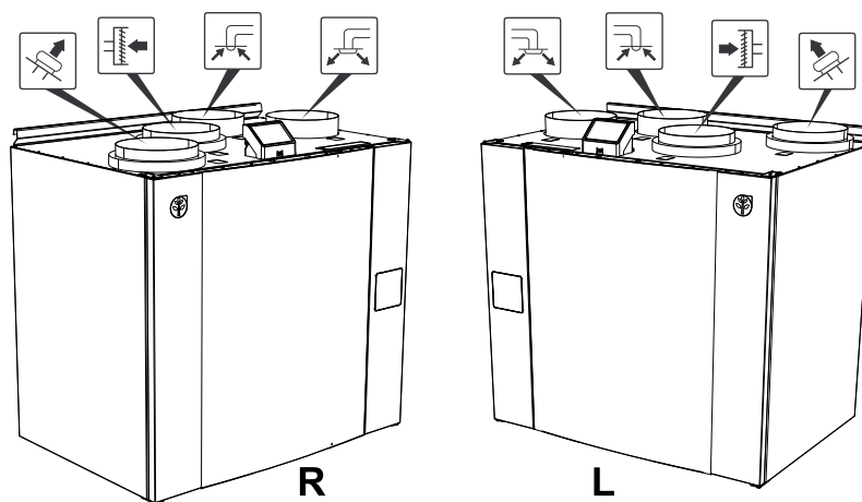
Bild 4 Kanalanschlüsse
